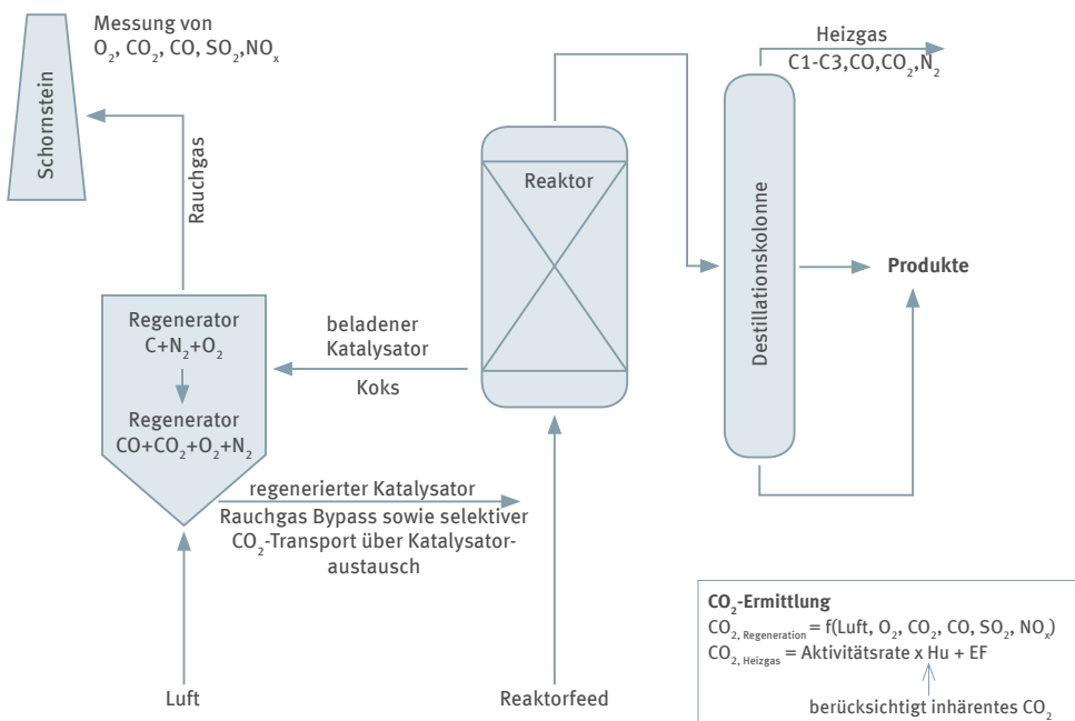
Abbildung 7: Schema der FCC-Anlage
