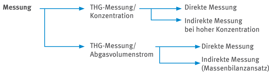
Abbildung 3: Varianten der kontinuierlichen Emissionsmessung
